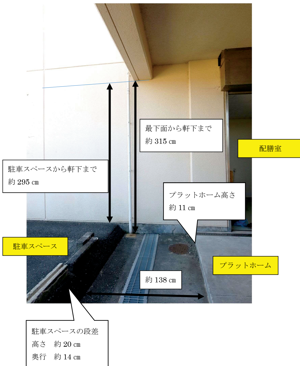
資料 7-4 小沢小学校 プラットホーム 断面・寸法
