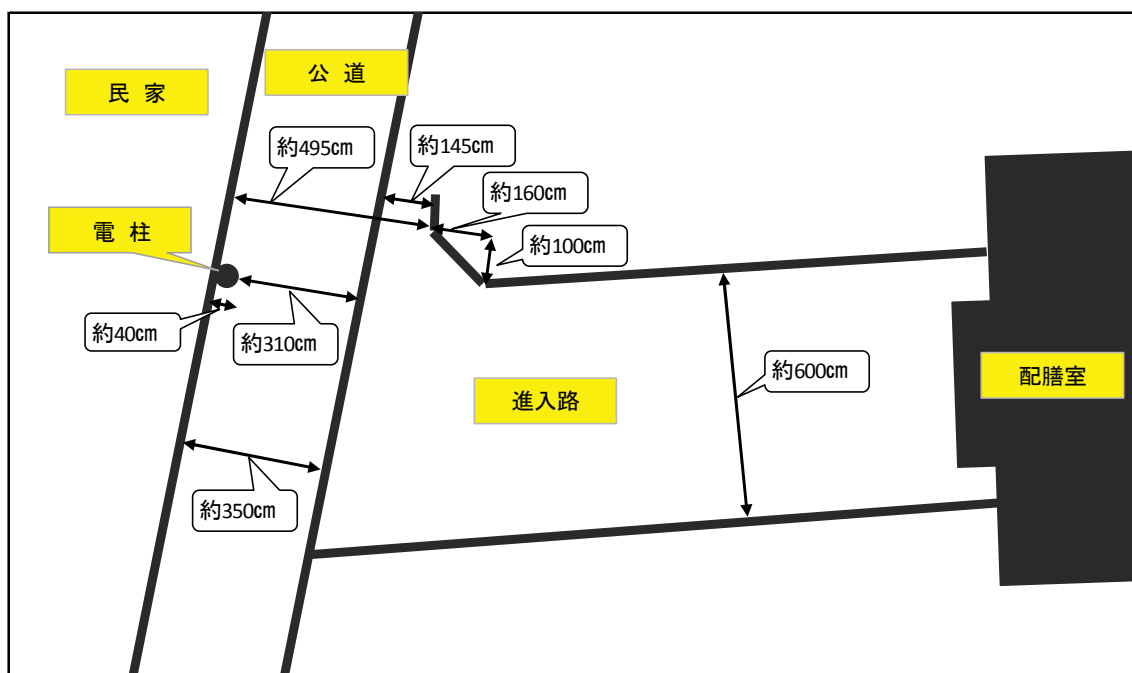
資料 7-3 旭小学校 配送車進入路
