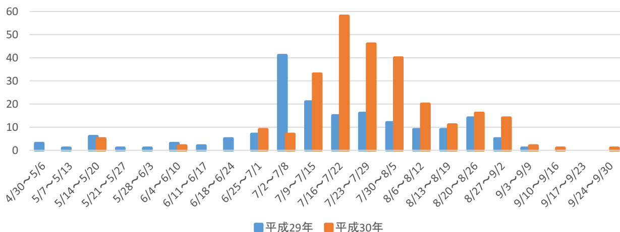
平成30年 熱中症による救急搬送者数 (昨年同時期との比較)
