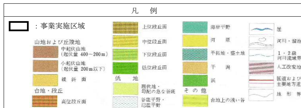
図 3-1-18 地形分類
