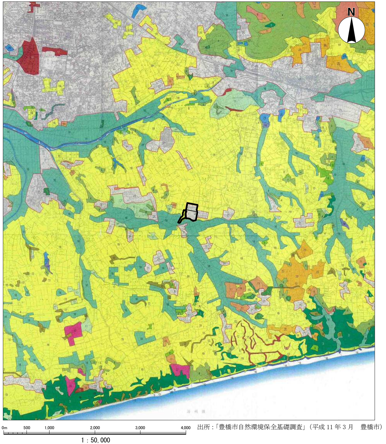
図 3-1-26 植生
