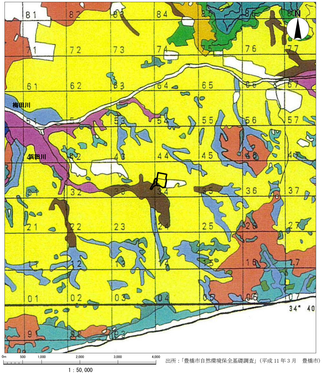
図 3-1-24 土壌
