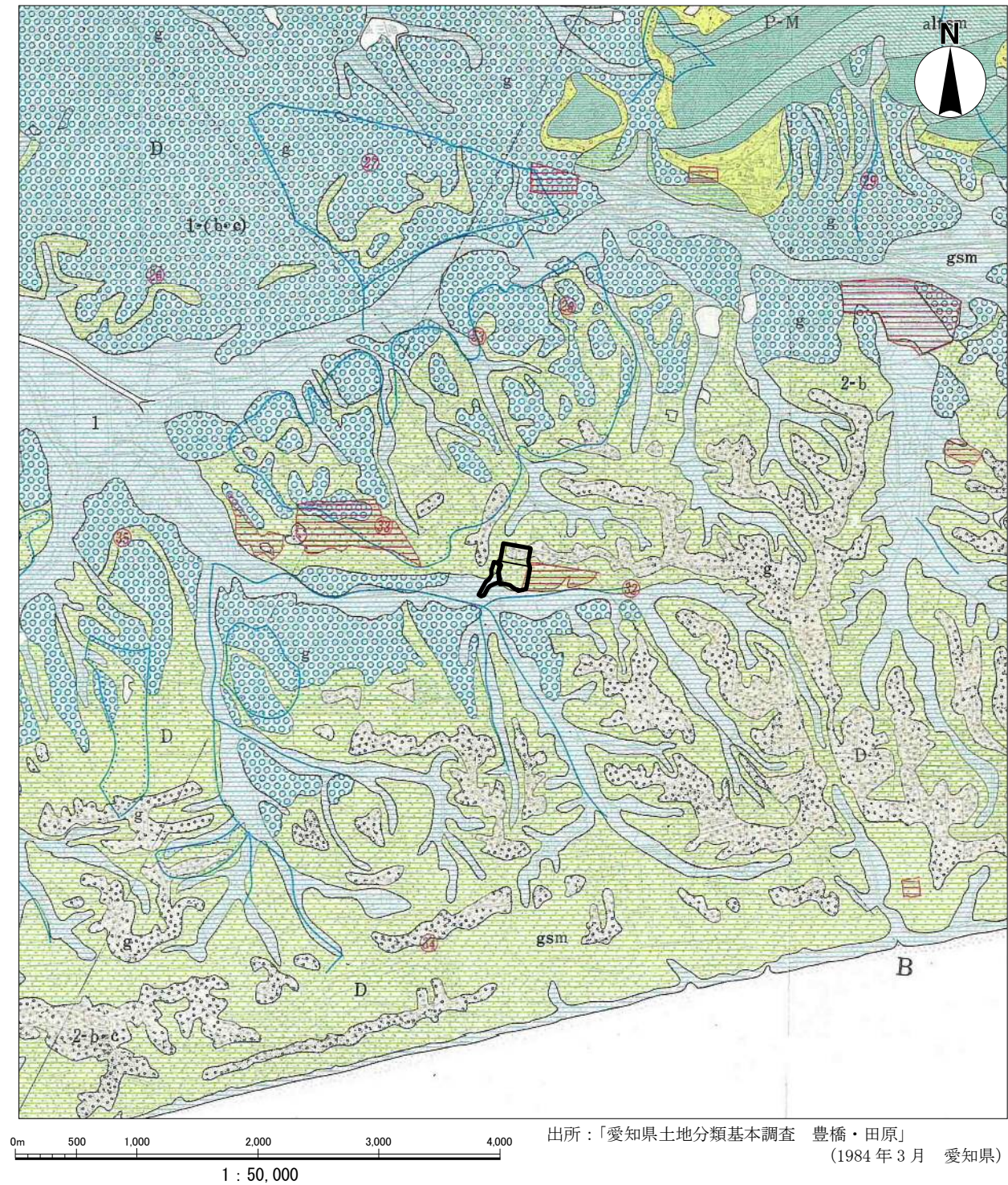
図 3-1-19 表層地質
