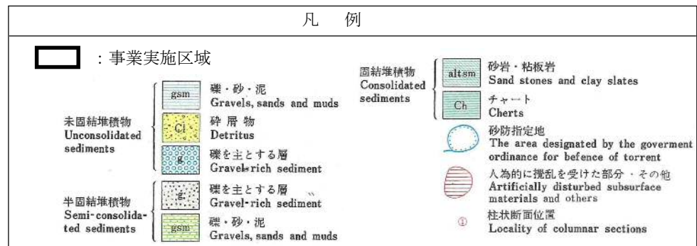
図 3-1-19 表層地質
