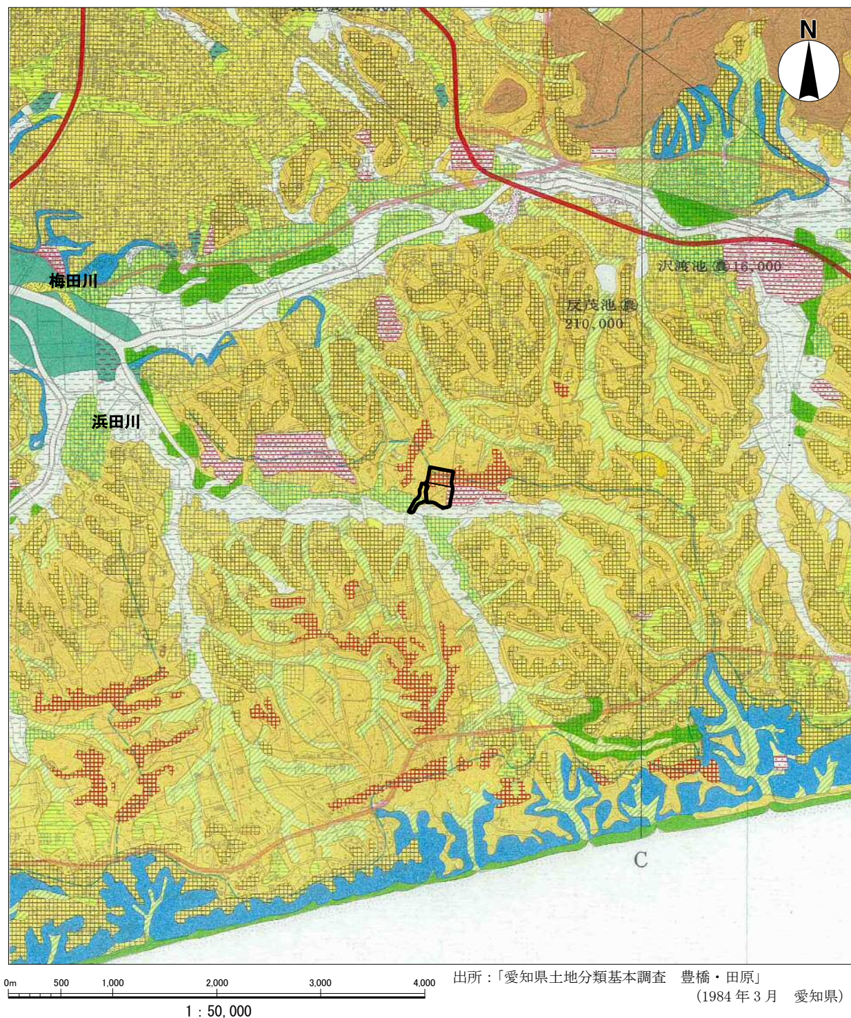
図 3-1-18 地形分類
