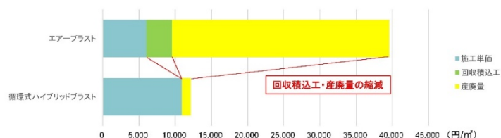
ブラスト工法の経済比較
