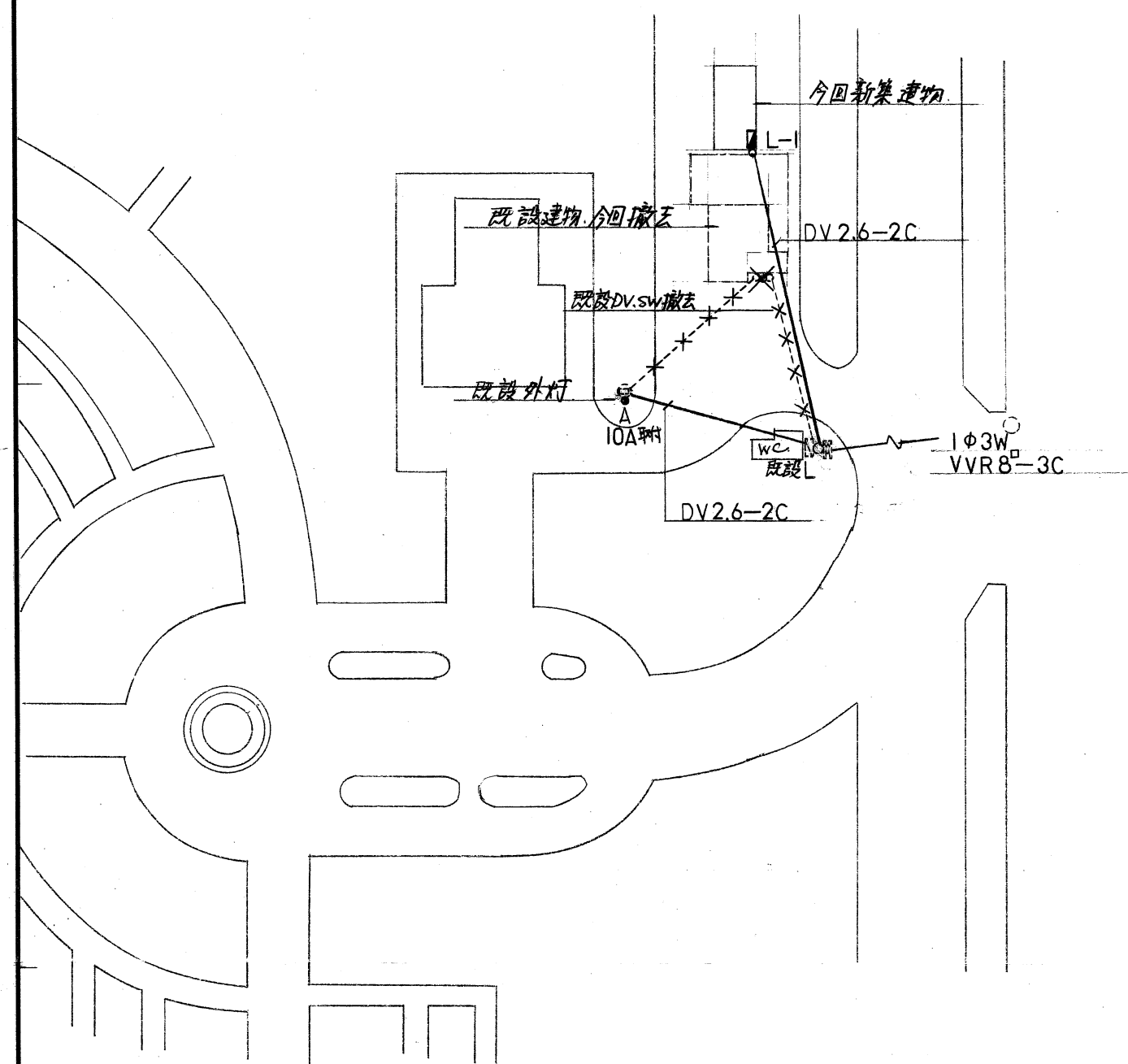
配置図 1:600
