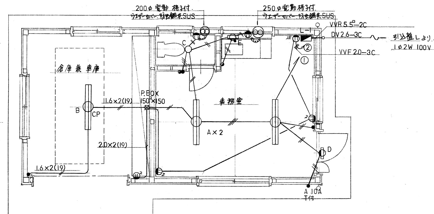
平面図 1:50
