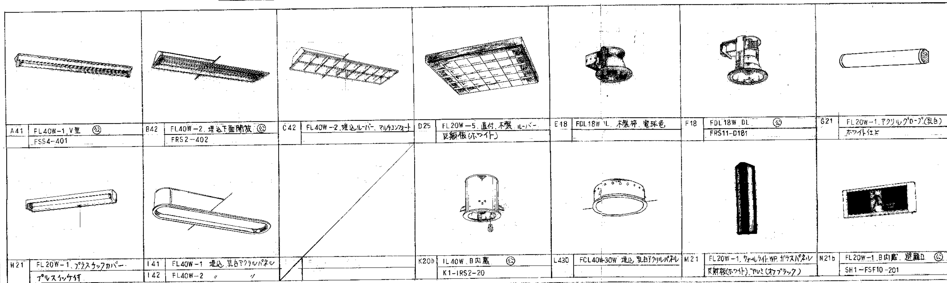
電灯設備平面図 1/100
