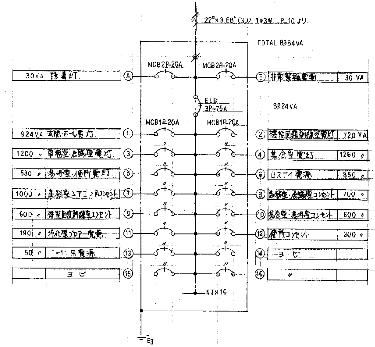
L-11 分電盤図 理込
