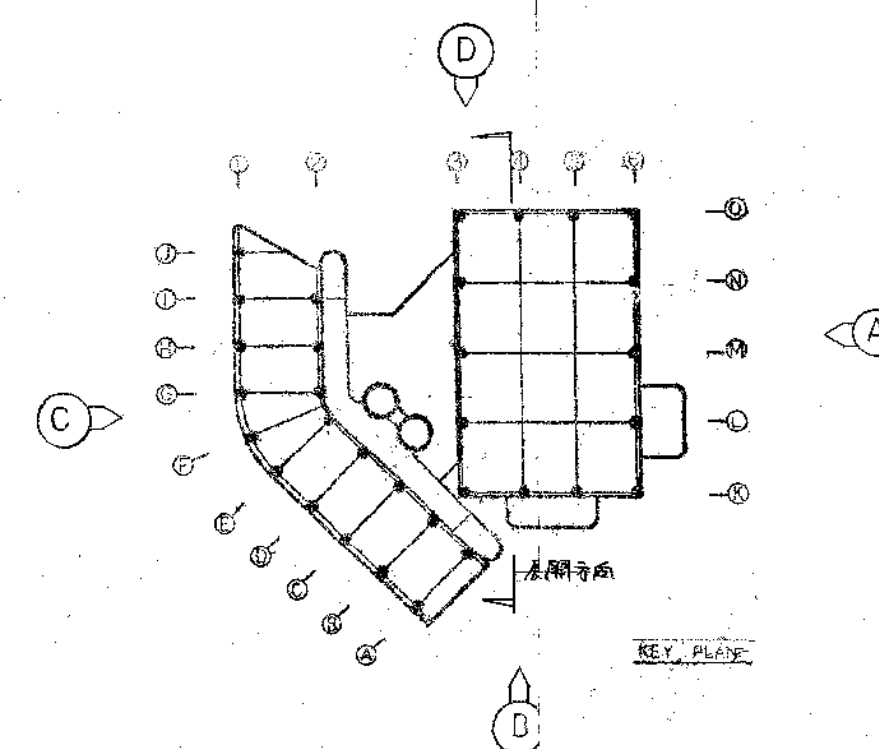
キープラン
