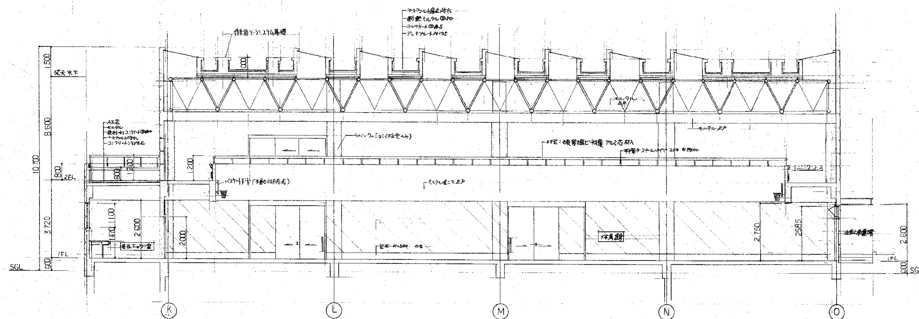
洋館 断面図
