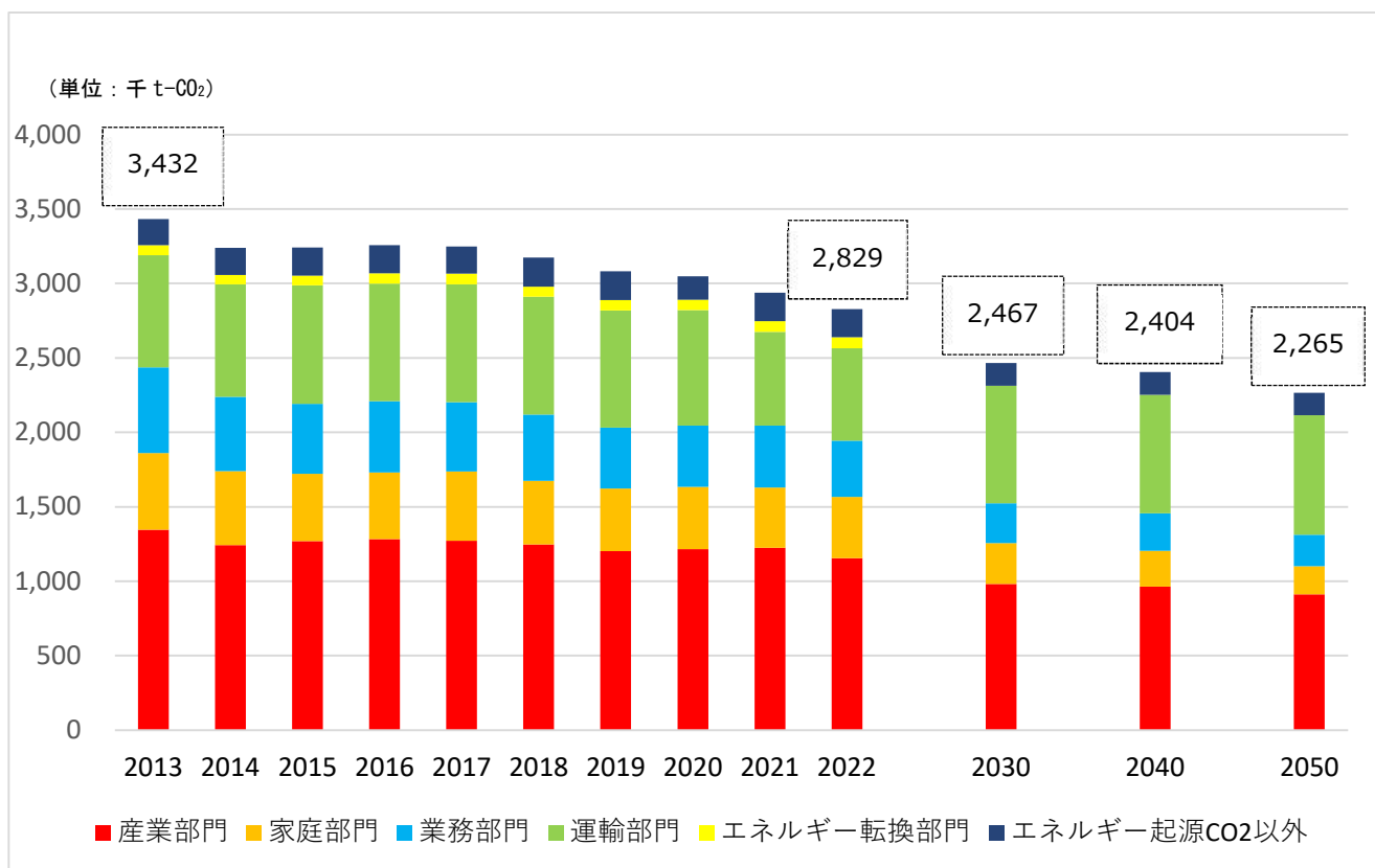
図3-4 温室効果ガス排出量の推計値
