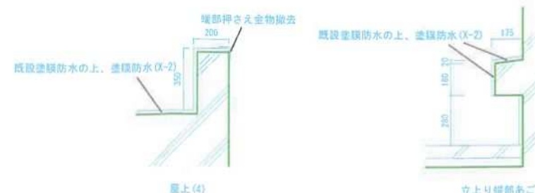
部分詳細図
