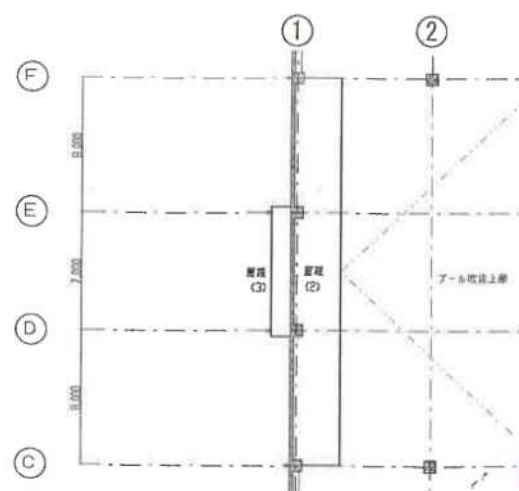
2階部分平面図 1/300
