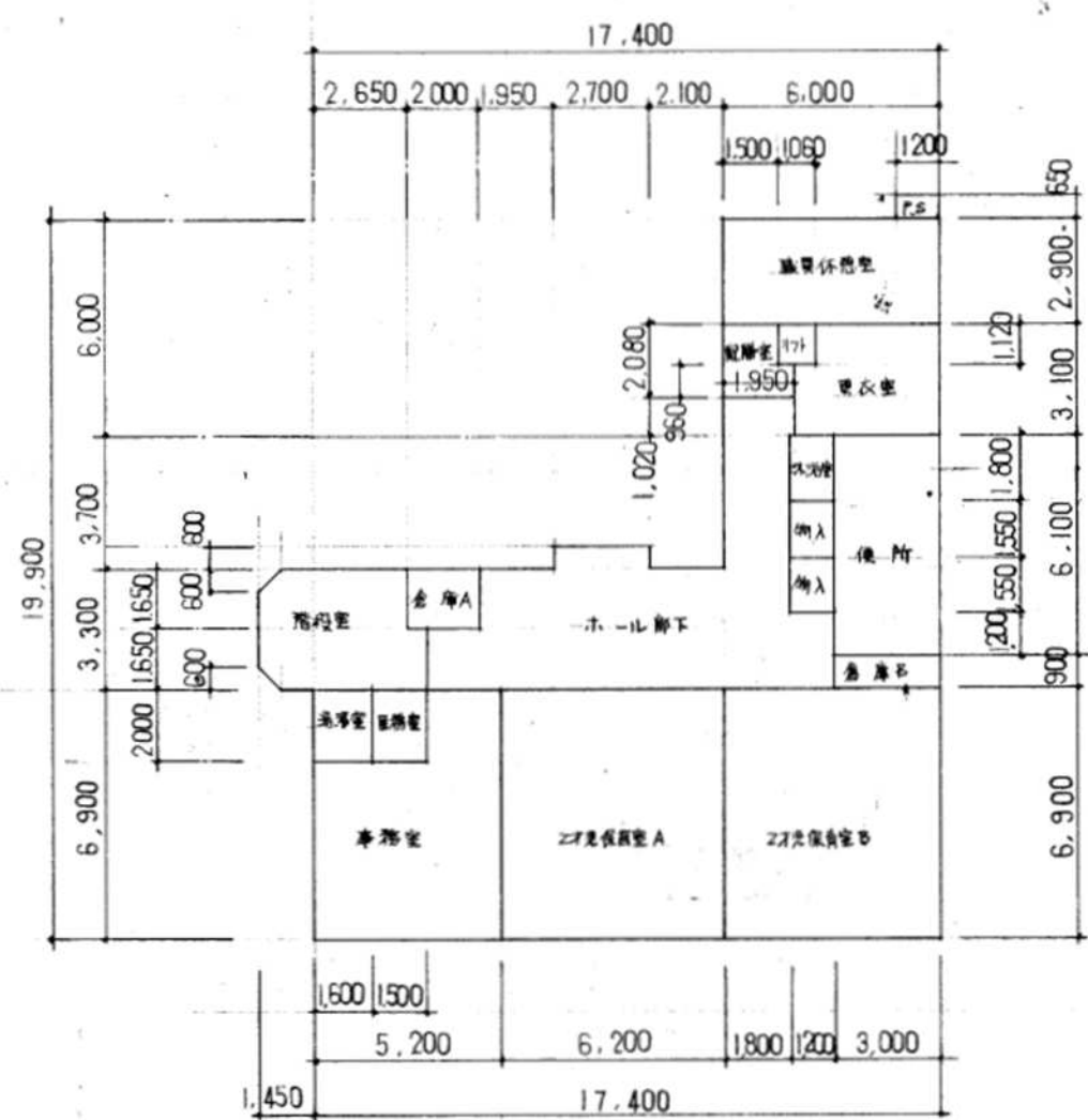
2 階平面図
