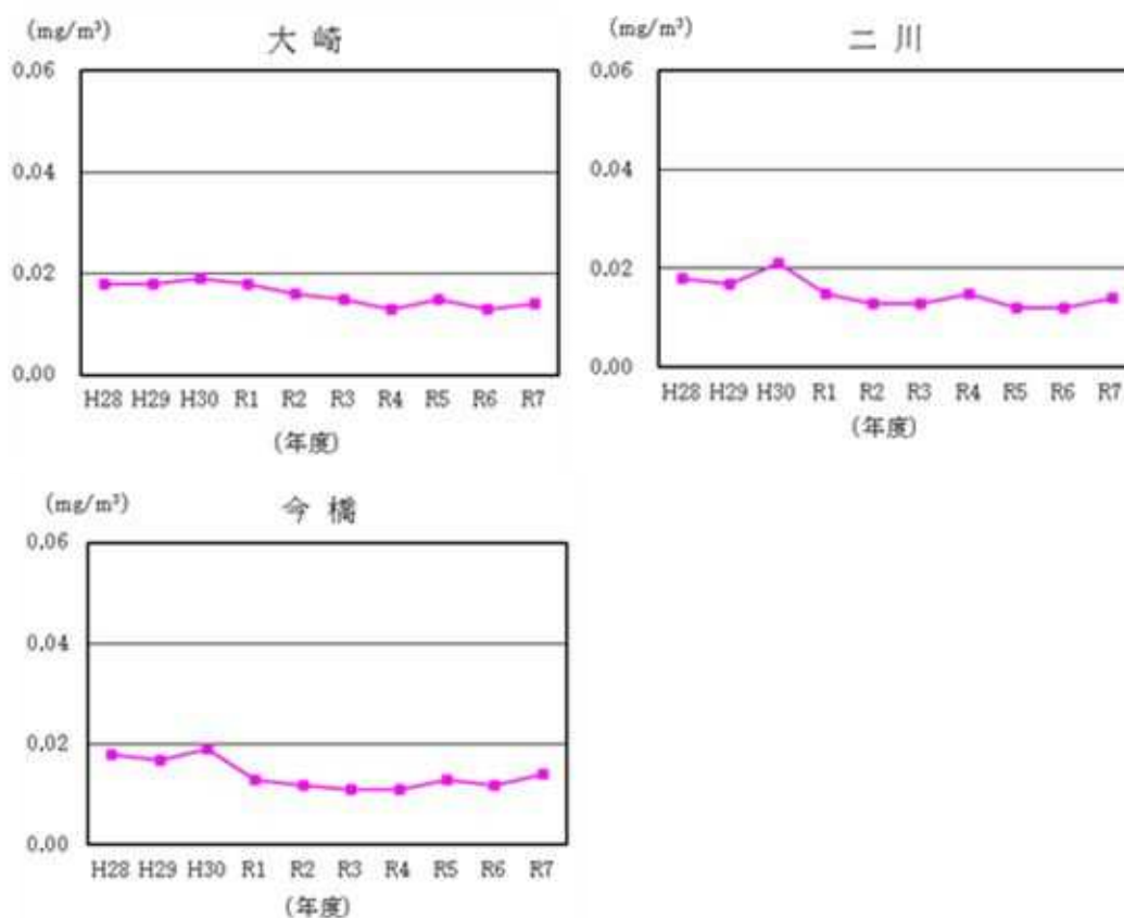
浮遊粒子状物質濃度の経年変化
