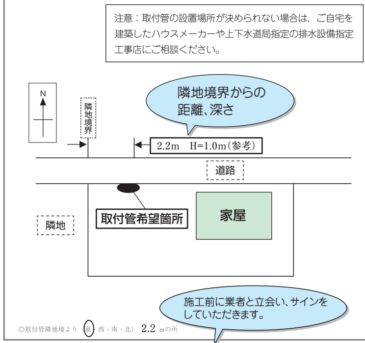
取付管設置希望位置詳細図
