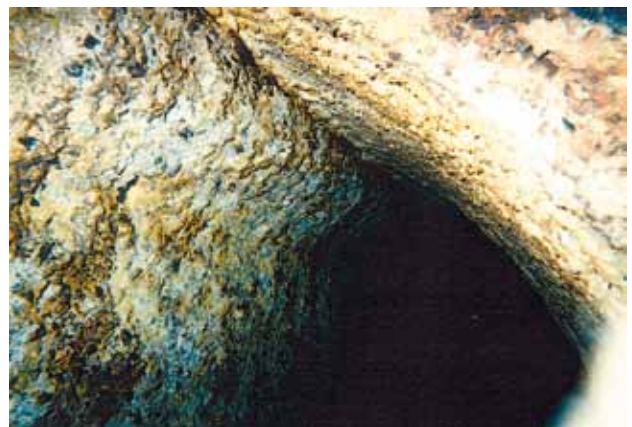
酸でぼろぼろになったコンクリート管 （下水道管：直径2m）
