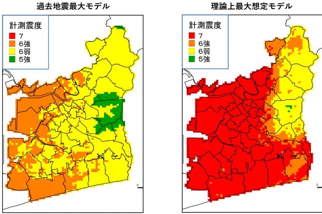
図 1-2 震度分布図
