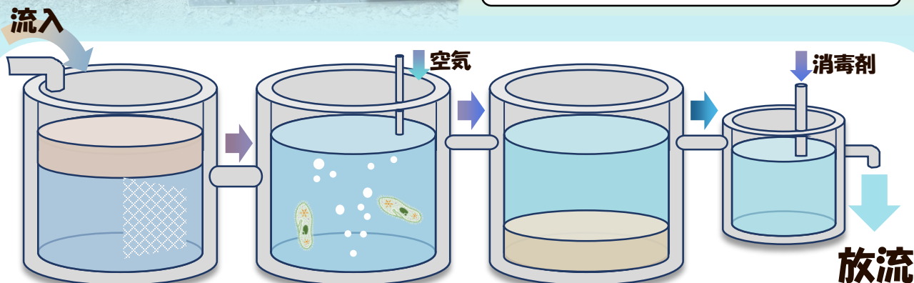
沈殿槽
