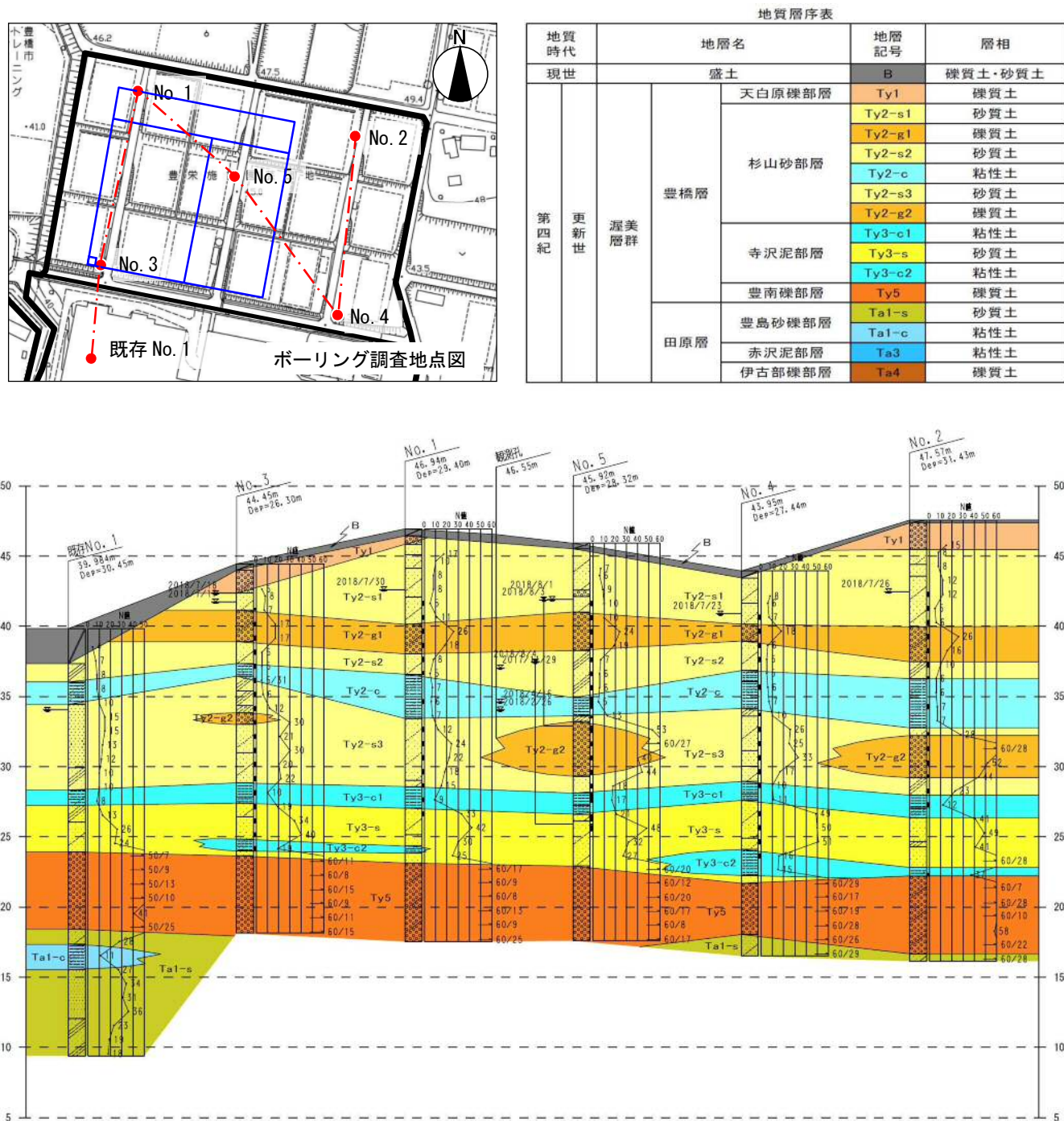
図 8-7-2 推定地層断面図
