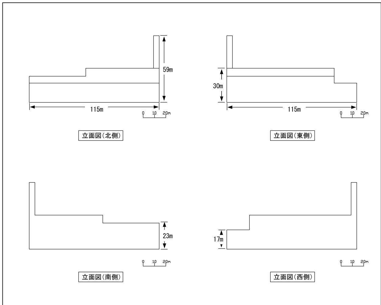
図 8-8-3 計画施設立面図
