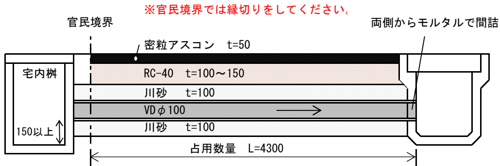
縦断面図（単位:mm）
