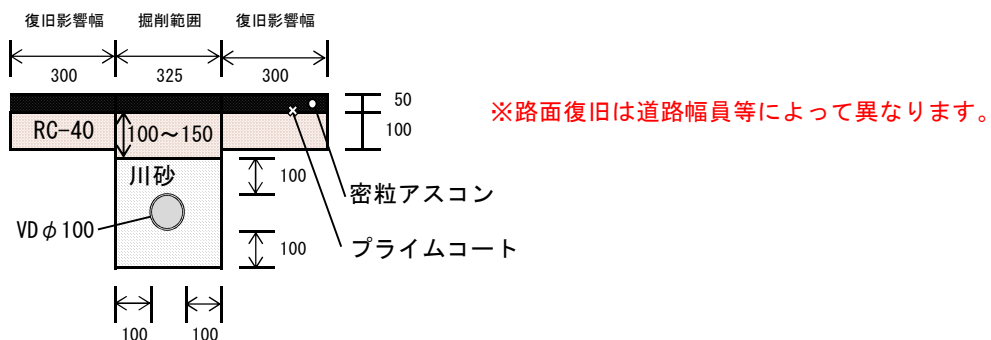
横断面図（単位:mm）
