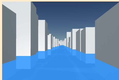
浸水シミュレーションのイメージ (PLATEAU VIEWより)
