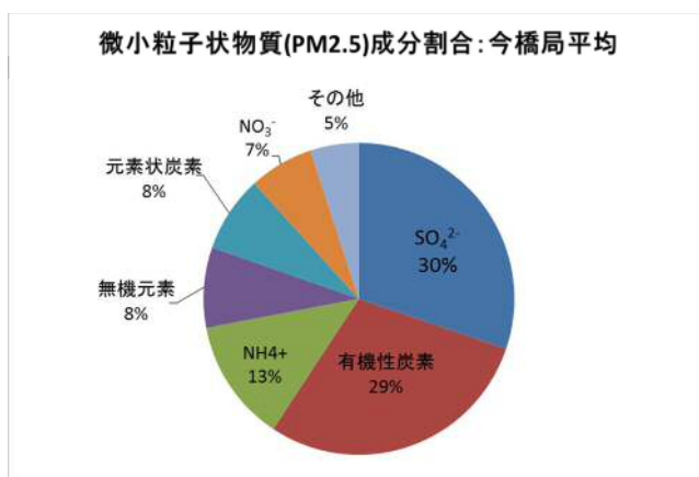
図 2 豊橋市内(今橋局)微小粒子状物質成分割合
