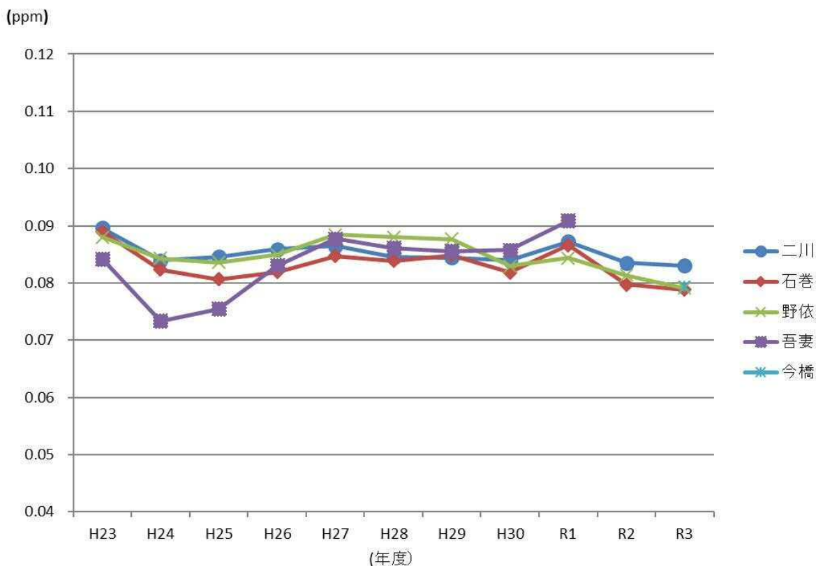
局ごとの日最高8時間値の年間99パーセンタイル値の3年移動平均値の経年変化
