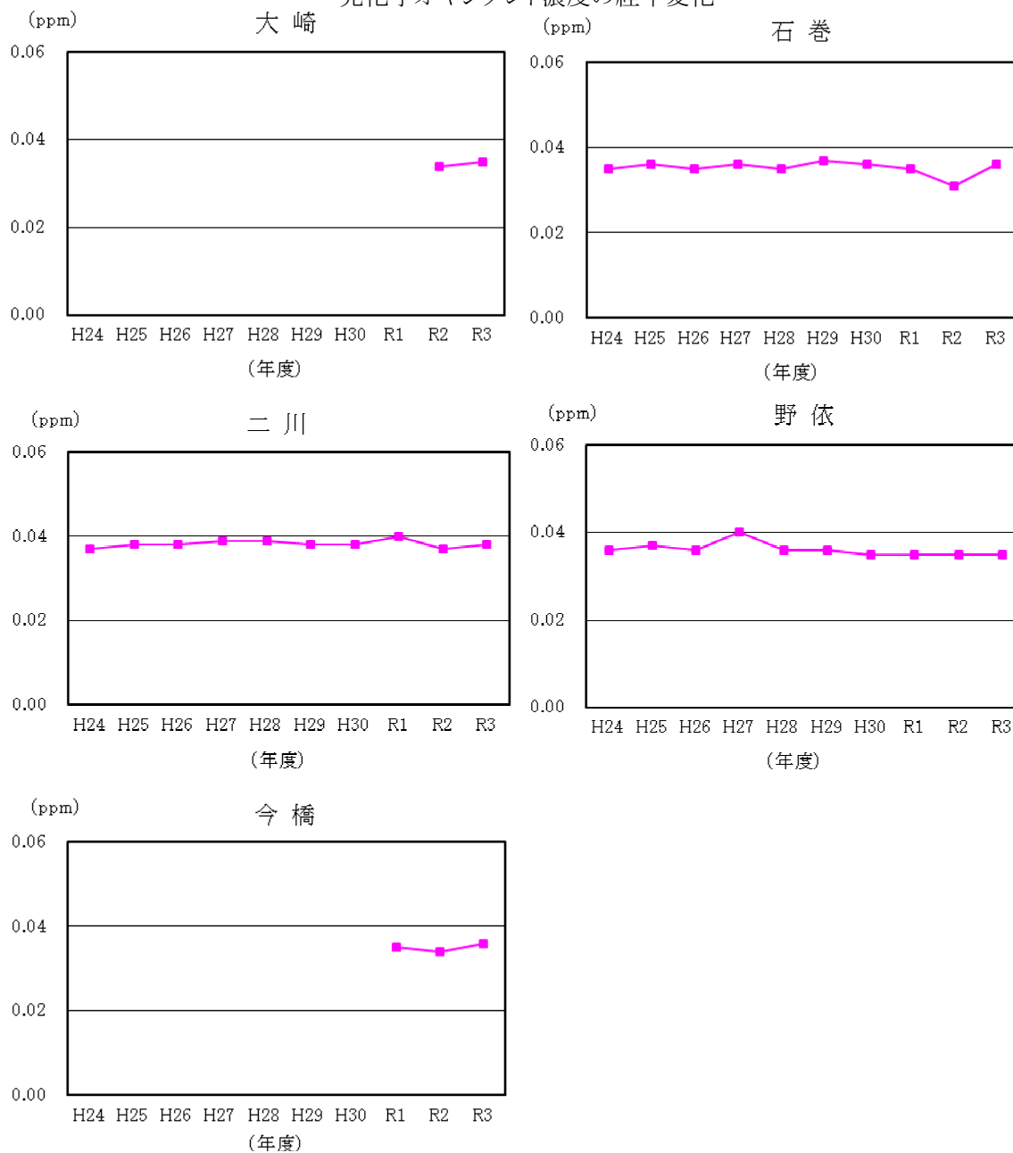
光化学オキシダント濃度の経年変化
