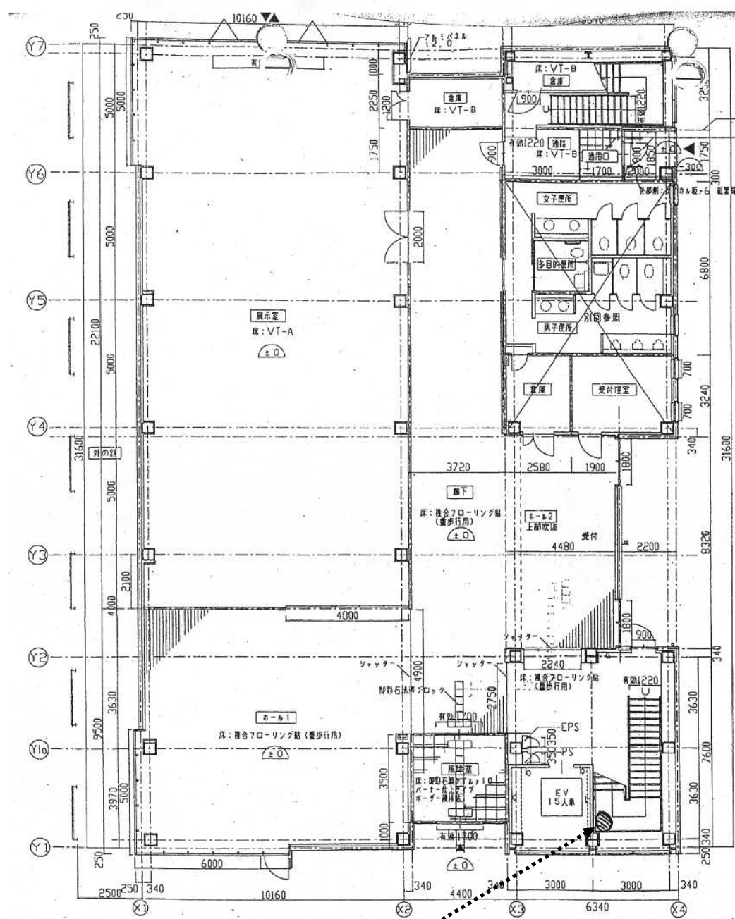
設置場所 平面図
